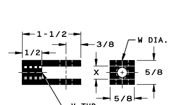
ROD CLEVIS
