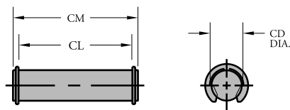
PIVOT PIN
